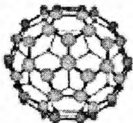
4.6-rasm. O'nlab atomlardan iborat uglerod molekulari.
