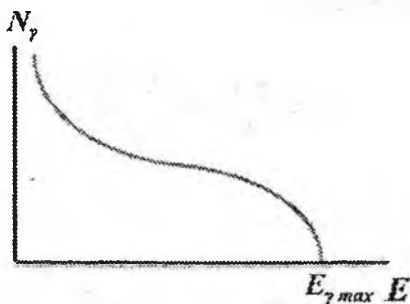
6.5-rasm. Tormozli nurlar spektri.
