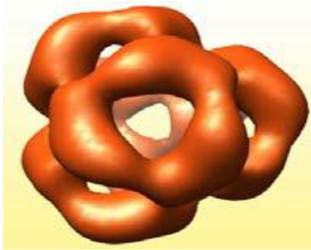
2-rasm. Oqsil molekulasini - tirik sistemada eng ko'p tarqalgan nanostrukturalari (kattaligi 4-50 nm).
