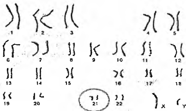
autosomes
