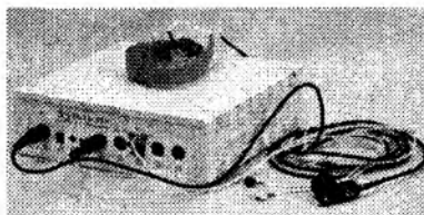
2.28-rasm. «SINAPSIS» rusumli to'rt kanalli elektromiografning umumiy ko'rinishi
