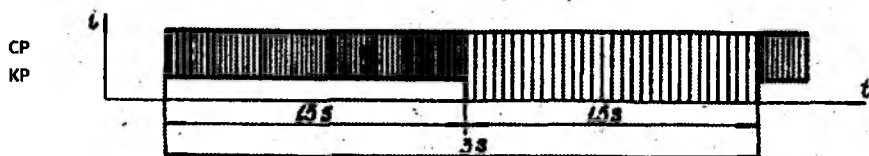
3.18-rasm. Qisqa davr (KP) - OH ko‘rinishidagi tok impulslari seriyasining DH ko‘rinishli tok impulslari seriyasi bilan almashinishi
