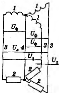
2.4-rasm. Uch fazali tok sistemasini ulash sxemasi: 1 – bitta generatorning faza o'ramlari, ularda o'zgaruvchan kuchlanish induktsiyalanadi; 2 – nagruzkalar (iste'molchilar); 3 – chiziqli simlar (ular generatorni iste'molchi bilan birlashtiradi); 4 – neytral (nol) simi
