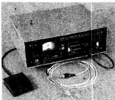
3.4-rasm. «EXVCh-20-01» YuCh elektroxirurgiya apparatining umumiy ko'rinishi
