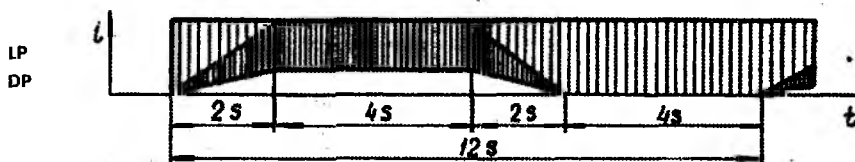
3.19-rasm. Uzoq (Uzun) davr (DP) – OH ko‘rinishidagi tok impulslar seriyasining almashinishi va DH ko‘rinishidagi tok impulslari seriyasigacha to‘ldirilishi egiluvchan bo‘lib, noldan to‘ OH ko‘rinishidagi tok amplitudasigacha ortadi, bu qiymatni ancha saqlab yana qaytib nolga tushishi mumkin.
