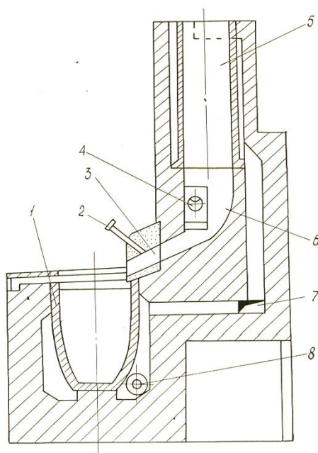
Shaxta-tigel pechi
