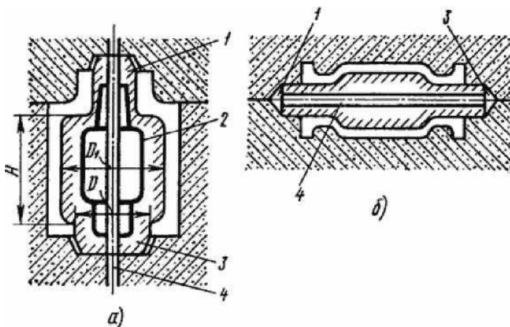
Rasm. 2. Uzaklarning belgisi: a — vertikal, b — gorizontal
