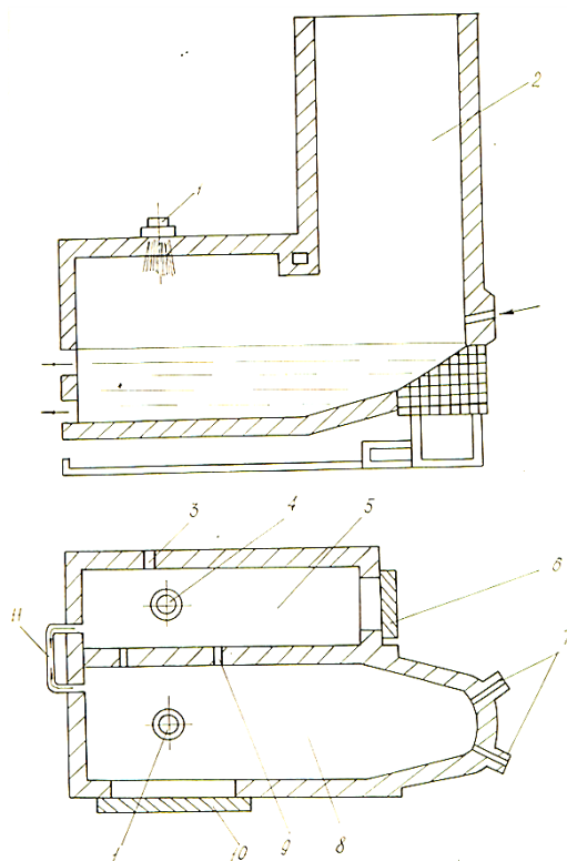
«Djet Melter» gaz qaytaruvchi pechi
