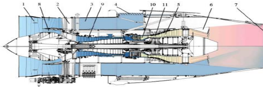
Рисунок 1.2.1.3_1 – Конструктивная схема ТРД (ПС-90А) 1 – вентилятор; 2 – раздельный корпус; 3 – канал наружного контура; 4 – реверс тяги; 5 – турбина вентилятора (низкого давления); 6 – смеситель; 7 – общее сопло; 8 – опорные ступени на валу вентилятора; 9 – компрессор высокого давления; 10 – камера сгорания; 11 – турбина высокого давления
