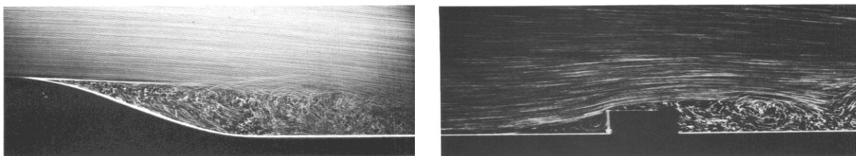
15 -rasm. Силлик (а) ва тўғри тўртбурчак (б) шаклидаги бўртиқ тўсиқларда
