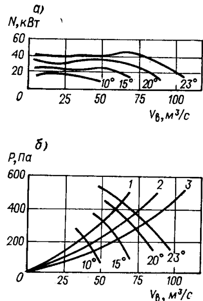
26-rasm. Aylanish chastotasi 7,5 \text{ s}^{-1} , AVG va ventilyatorlarning aerodinamik xarakteristikalari a-iste'mol kuvvati; b-AVG karshiligi (katorlar soni 1 da – 8; 2 da – 6; 3 da – 4)
