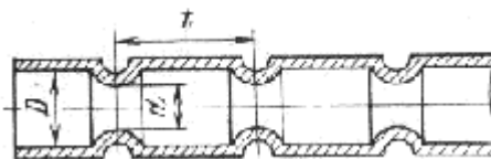
16 - rasm. Tashqi tomonida kўndalang botiq ariqcha va ichki tomoni sillik бўртиқ тўсиқли самардор иссиқлик алмашиниш юзаси.
