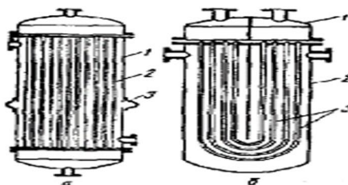
6 - rasm. Xarorat kuchlanishlarini kompensatsiya qiluvchi issiqlik almashinish qurilmasining tuzilishi: a) linza kompensatorli: 1- qobiq; 2- isituvchi Quvur; 3- linzali kompensator. b) U-simon Quvurli: 1- qopqoq; 2 -qobiq koplama; 3 -U-simon isituvchi Quvurlar.
