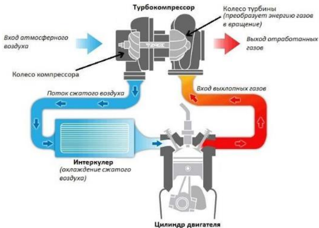
9-рasm. Турбонаддув тизими: турбина дарча билан ва компрессор.
