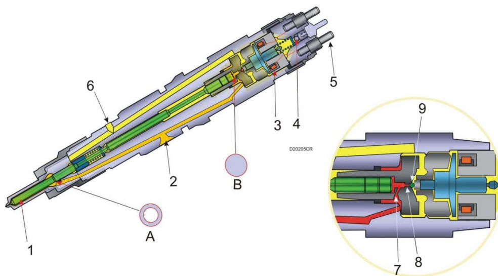
6-rasm. Pyezoelementli forsunka
