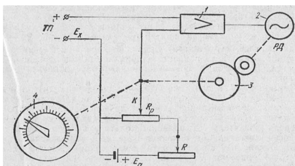
3.15- rasm. Elektron avtomatik potensiometrning tuzilish sxemasi.
