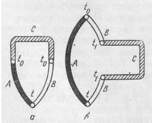
3.7-rasm. Uchinchi o'tkazgichni ulash sxemasi: a – termopara kavsharida zanjirni uzish; b – termoelektrodlardan
