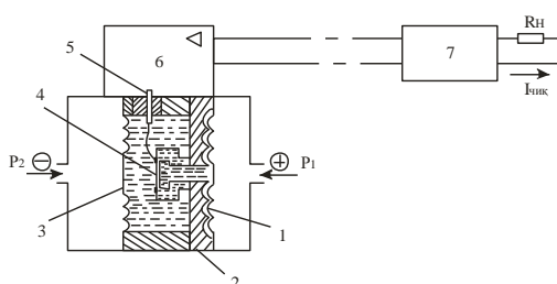
4.18 – rasm. Sapfir – 22 DD-YEX bosimlar farqini o'lchovchi o'zgartkichning sxemasi.
