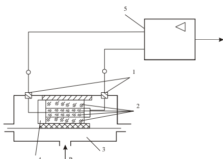
4.19 – расм. Пьезоэлектрик манометр схемаси
