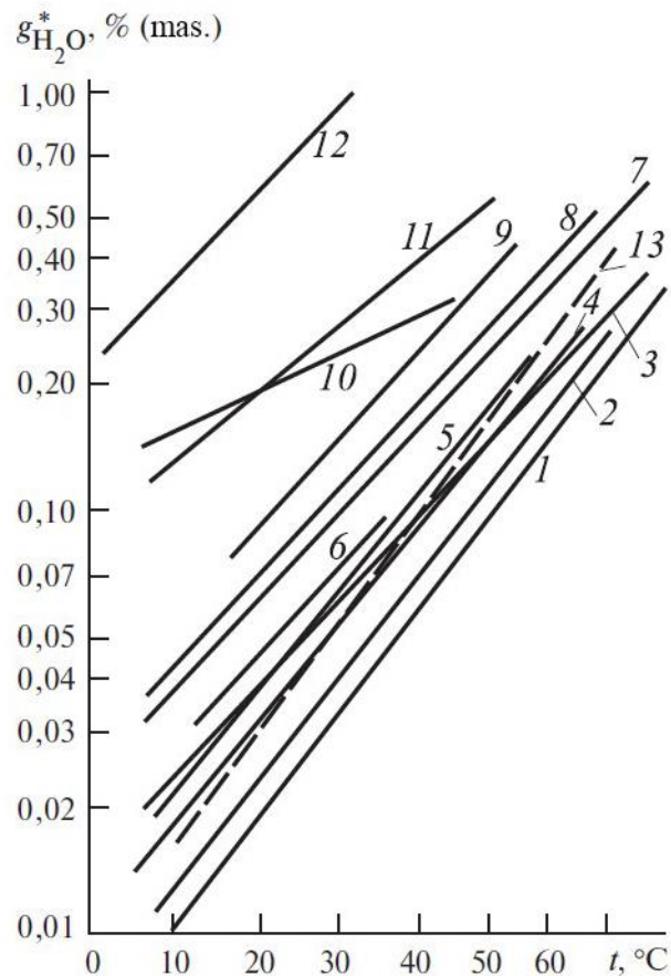
2.3-rasm. 0.101 MPa da suyuqlashtirilgan va suyuq uglevodorodlarda suv yeruvchanligining haroratga bog‘liqligi: 1 – n-butan; 2 – izobutan; 3 – propan; 4 – n-pentan; 5 – izopentan; 6 – siklogeksan; 7 – n-geksan; 8 – n-geptan; 9 – n-oktan; 10 – butadien-1,3; 11 – benzin; 12 – gepten-1; 13 – SHFLU (engil uglevodorodlarning keng fraktsiyasi) (Nijnevartovsk GQZ)
