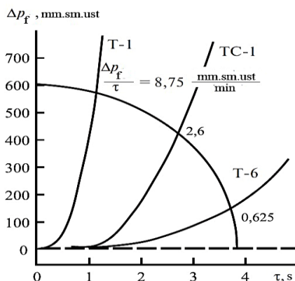
4.1-rasm. Harorat 165 °C da filtrda bosim \Delta p_f pasayishining yonilg'i haydalishi davomiyligiga bog'liqligi: sarjali to'qilgan filtr, yacheykalar o'lchami 12-16 mkm; reaktiv yonilg'ilar markalari – T-1, TS-1 va T-6.
