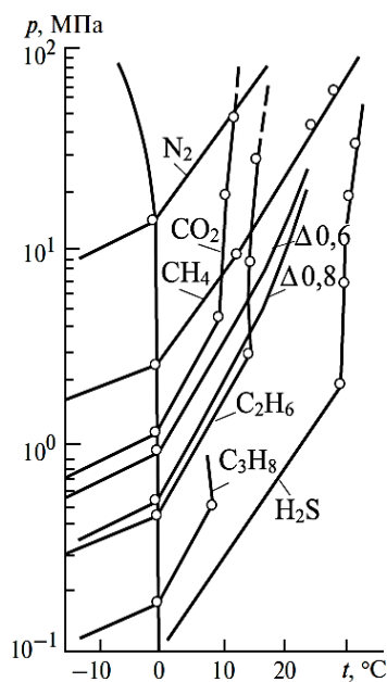
2.5-rasm. Xar xil zichlikdagi individual va tabiiy gazlarning giratlari hosil bo'lishining harorat va bosim bo'yicha muvozanatli shartlari: \Delta 0,6 va \Delta 0,8 - havo bo'yicha nisbiy zichlik
