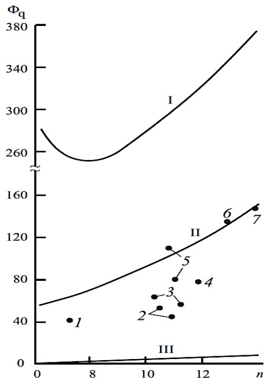
4.5-rasm. Alkil zanjirlari normal tuzilgan uglevodorodlar va benzinlarning molekularidagi atomlar soni p ga sohta omilining \Phi_s bog'liqligi: I — aromatik uglevodorodlar; II — naftenli uglevodorodlar; III — parafinli uglevodorodlar; 1 — benzin B-70; 2 — RT; 3 — TS-1; 4 — T-8V; 5 — T-1; 6 — T-6 ( TU 38.101629-82); 7 — T-6 ( GOST 12308-89)
