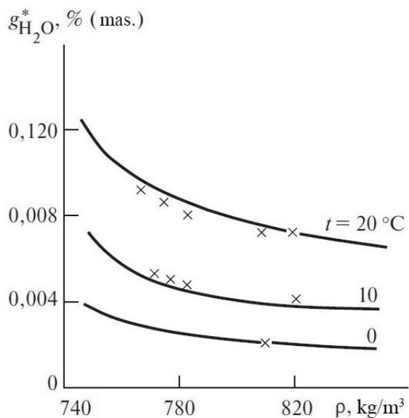
2.2-rasm. Havoning 100% nisbiy namligida yonilg'i zichligiga qarab suvning maksimal eruvchanligi
