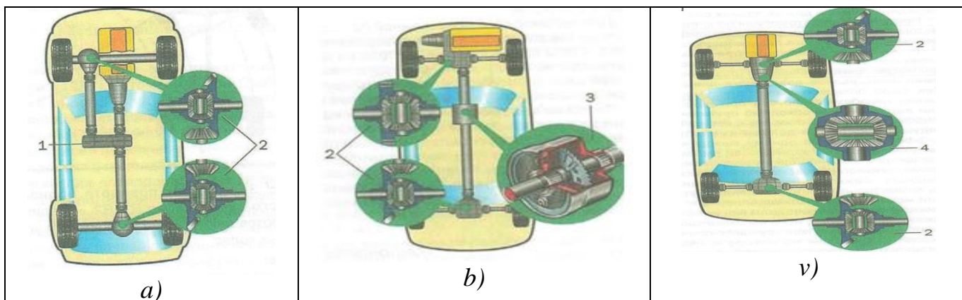
3.22-rasm. To'la yuritmalii transmissiyalar sxemalari: a-tarqatish reduktoriga ega (haydovchi qo'shadi); b-avtomatik viskomufta yordamida qo'shiladigan to'la yuritma; v-doimiy qo'shilgan to'la yuritma; 1-taqsimlash qutisi; 2-g'ildiraklararo differensial; 3- viskomufta; 4-o'qlararo differensial
