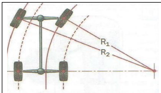
3.21-rasm. To'la yuritmalii avtomobil burilish sxemasi: R_1, R_2 – boshqariluvchi ichki va tashqi g'ildiraklar burilish radiuslari
