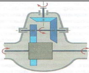
3.10-rasm. Ikkilangan bosh uzatma
